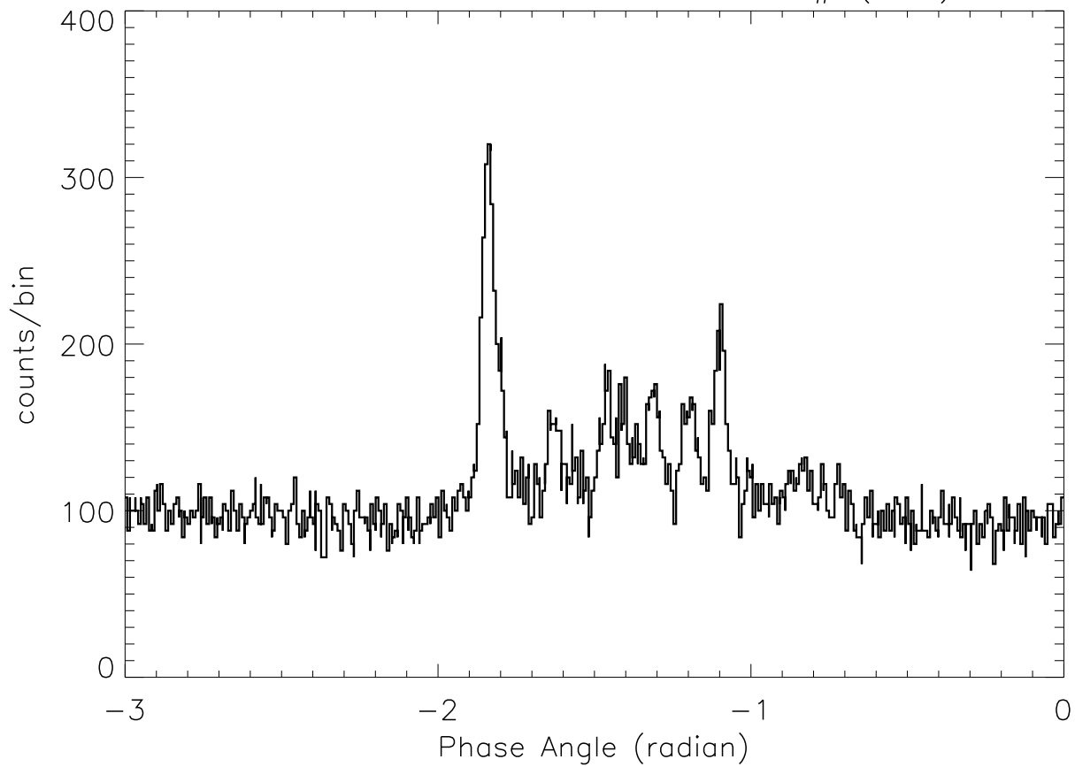
SOX2: 23: 1:26 – 23: 1:35 SP# ( 49)
