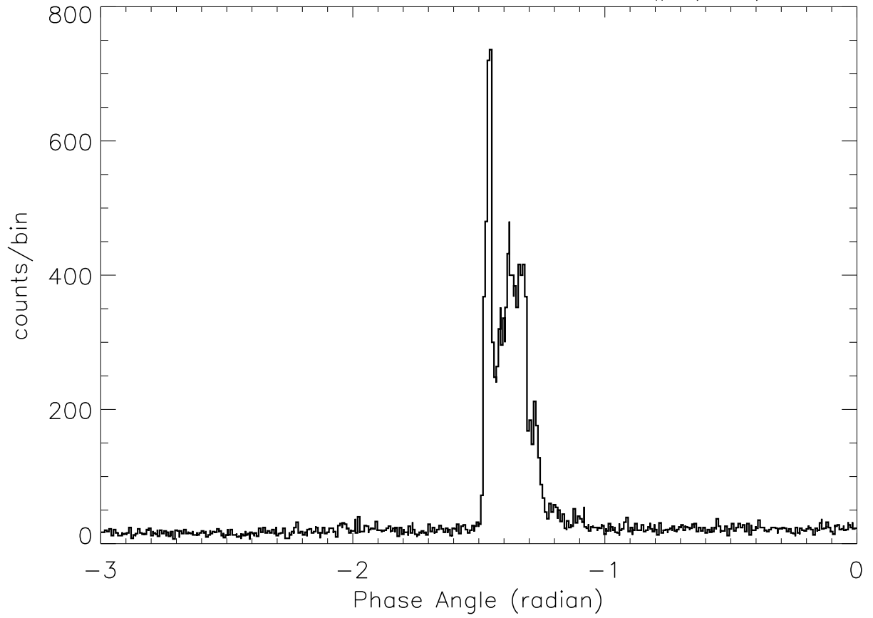
SOX2: 4:35: 6 – 4:35:14 SP# ( 26)
