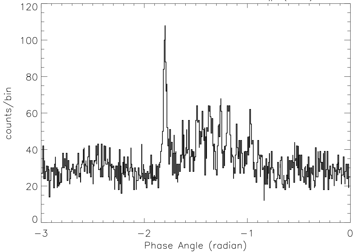
SOX2: 4:38:19 – 4:38:28 SP# ( 48)
