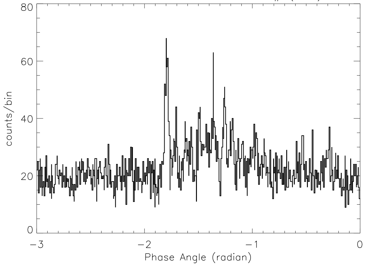
SOX2: 4:39:21 - 4:39:29 SP# ( 55)
