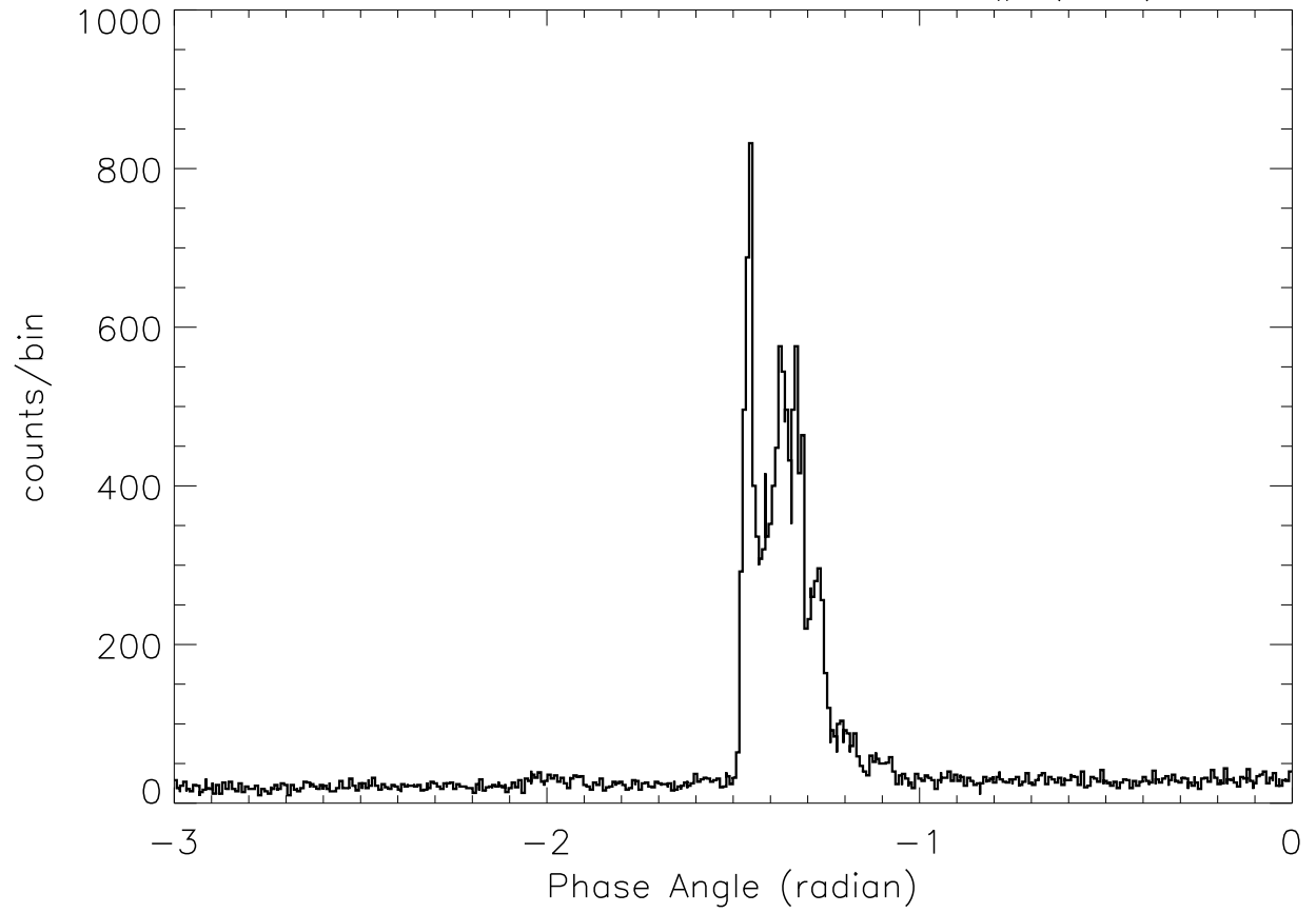
SOX2: 4:36:25 - 4:36:34 SP# ( 35)
