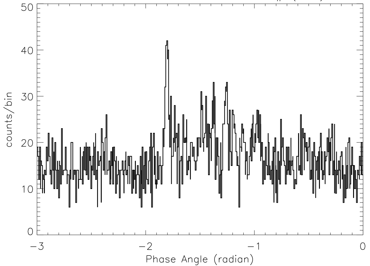
SOX2: 4:40:13 – 4:40:22 SP# ( 61)
