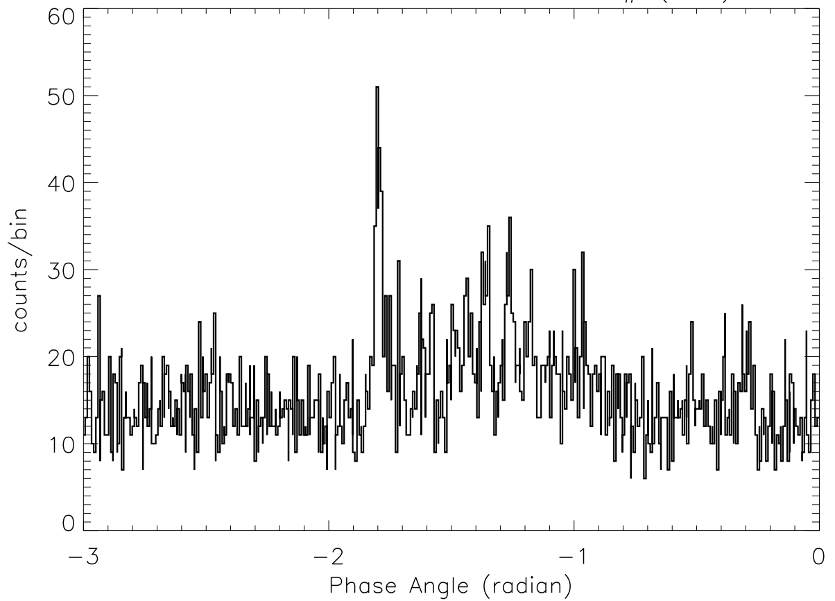
SOX2: 4:40:22 - 4:40:31 SP# ( 62)
