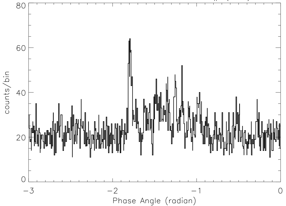
SOX2: 4:39:12 – 4:39:21 SP# ( 54)
