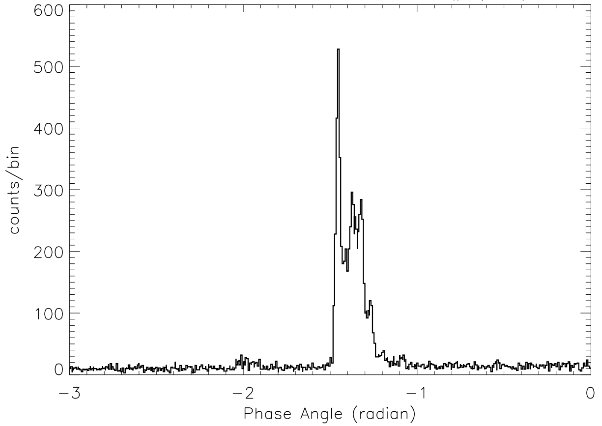
SOX2: 4:34:13 – 4:34:22 SP# ( 20)
