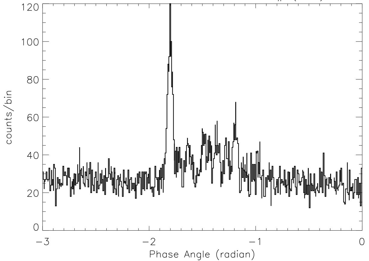
SOX2: 4:34:39 – 4:34:48 SP# ( 23)
