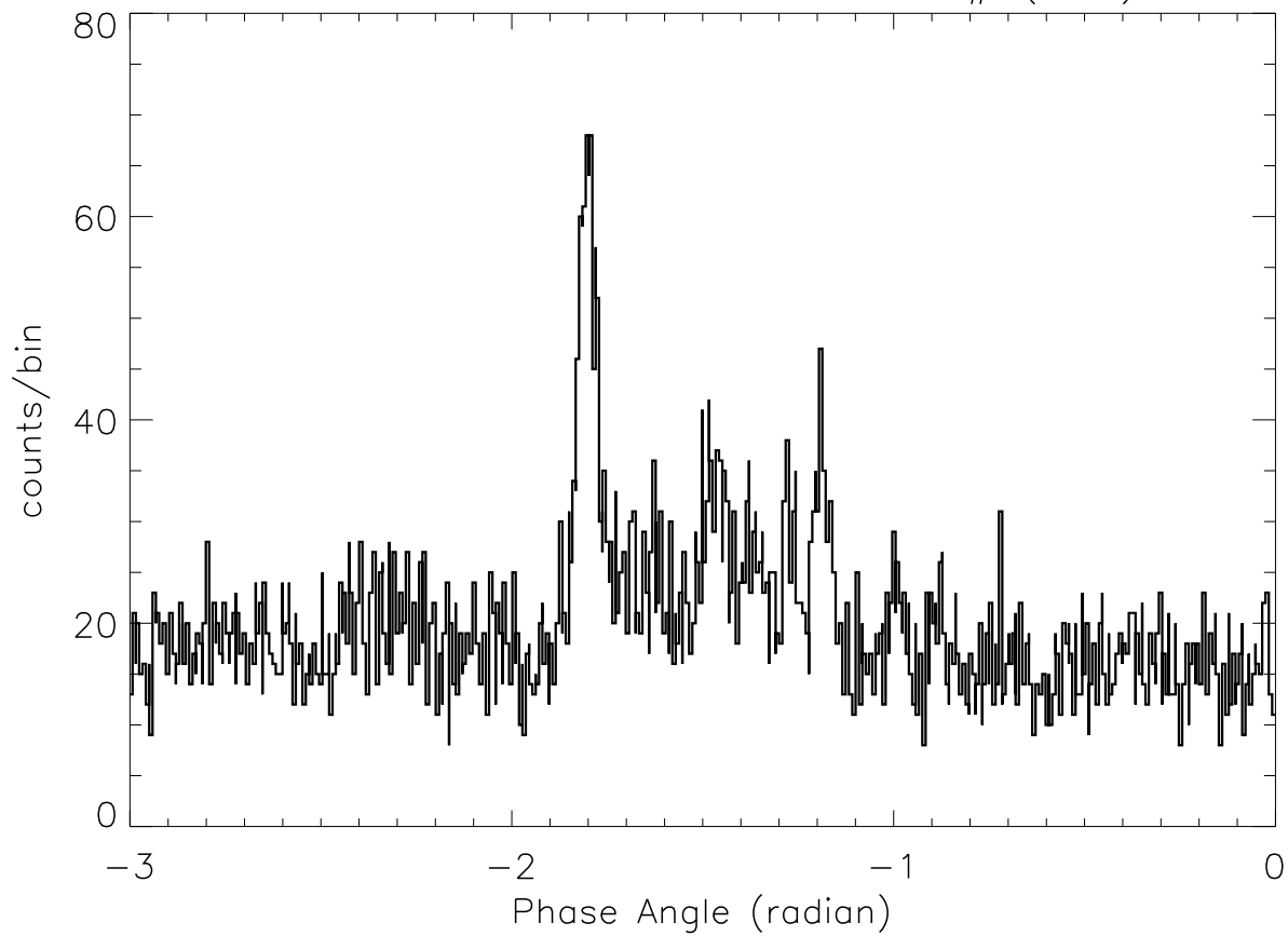
SOX2: 4:34: 4 - 4:34:13 SP# ( 19)
