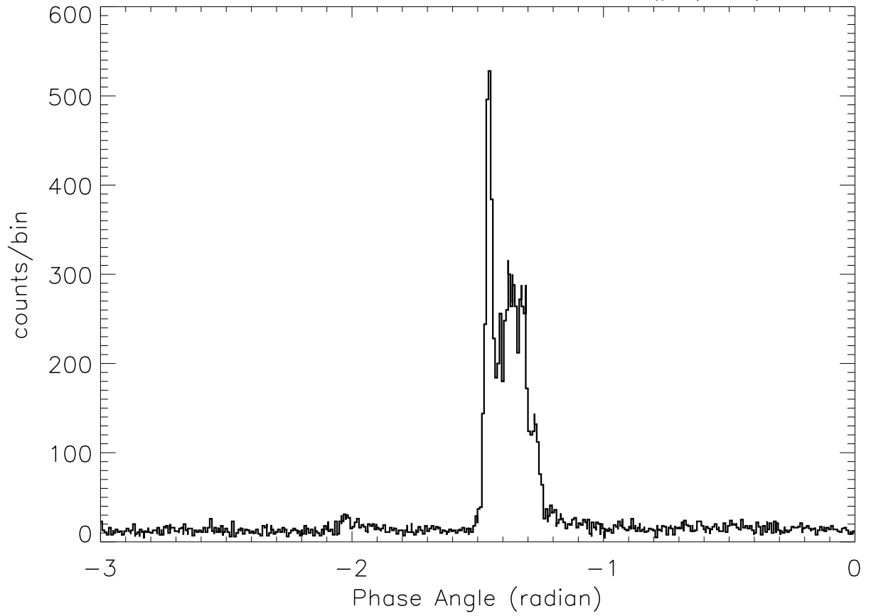
SOX2: 4:34:22 – 4:34:30 SP# ( 21)
