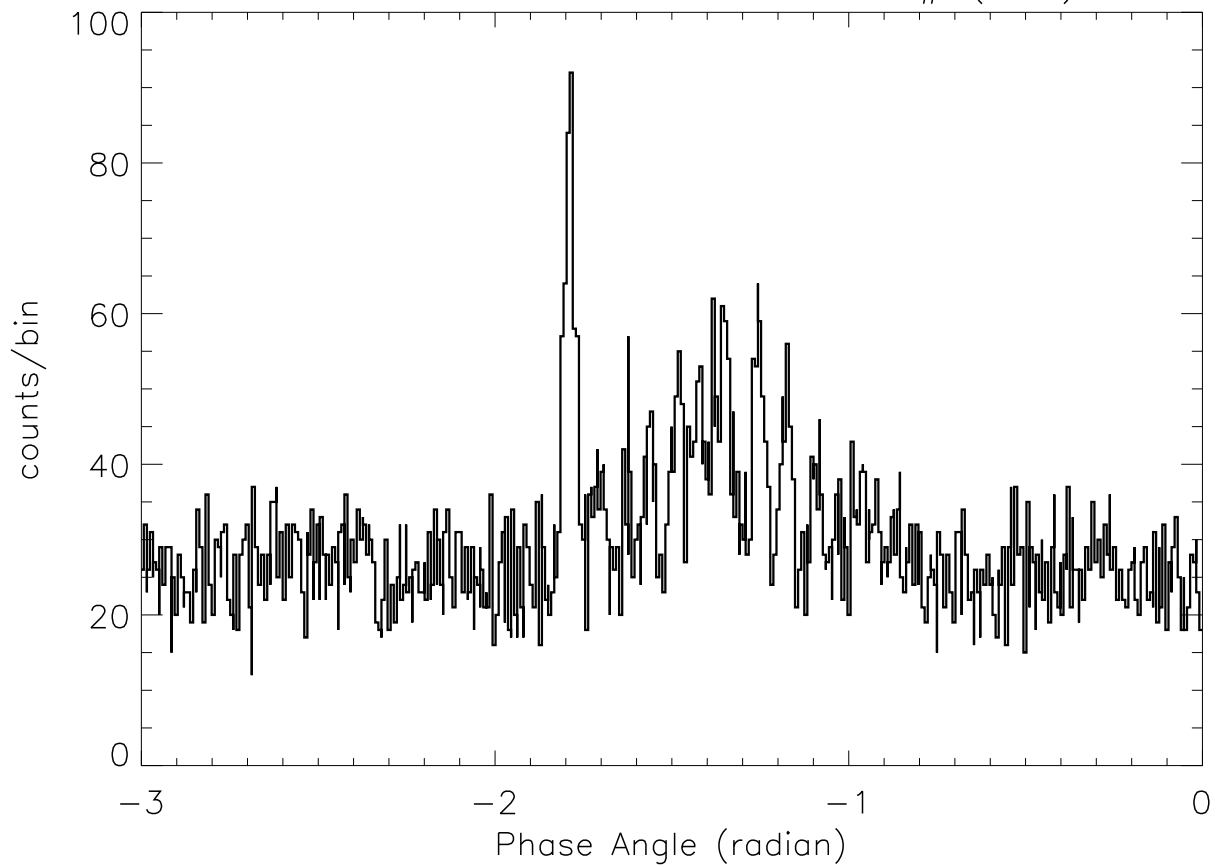
SOX2: 4:38:37 – 4:38:45 SP# ( 50)
