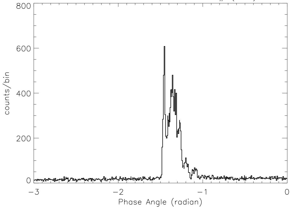
SOX2: 4:38: 1 - 4:38:10 SP# ( 46)
