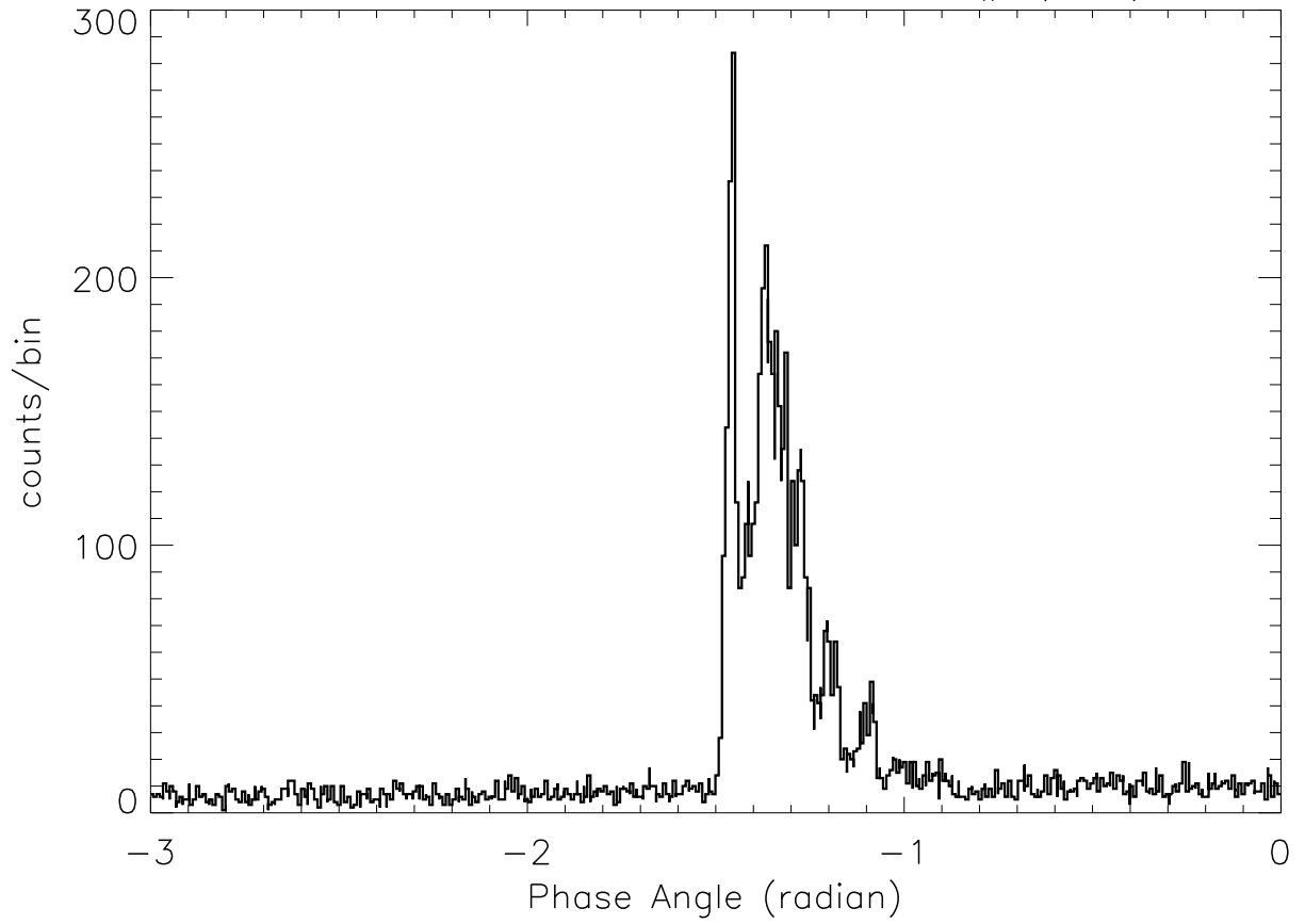
SOX2: 4:40:13 – 4:40:22 SP# ( 61)
