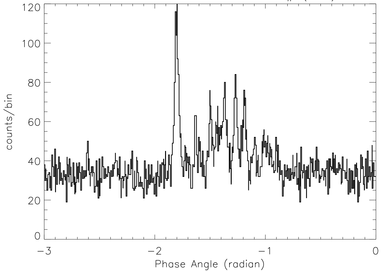
SOX2: 4:37:53 – 4:38: 1 SP# ( 45)
