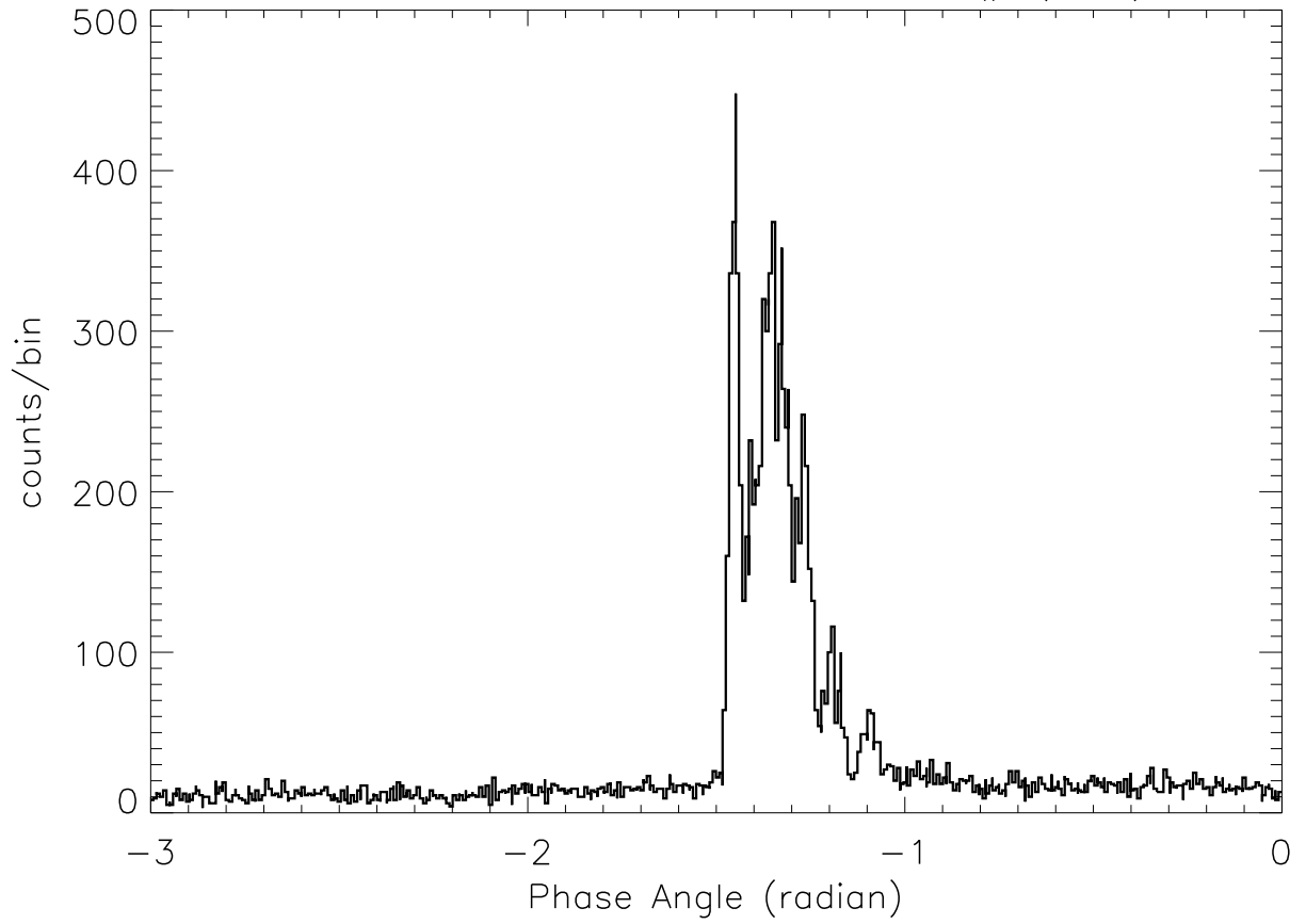
SOX2: 4:38:45 - 4:38:54 SP# ( 51)
