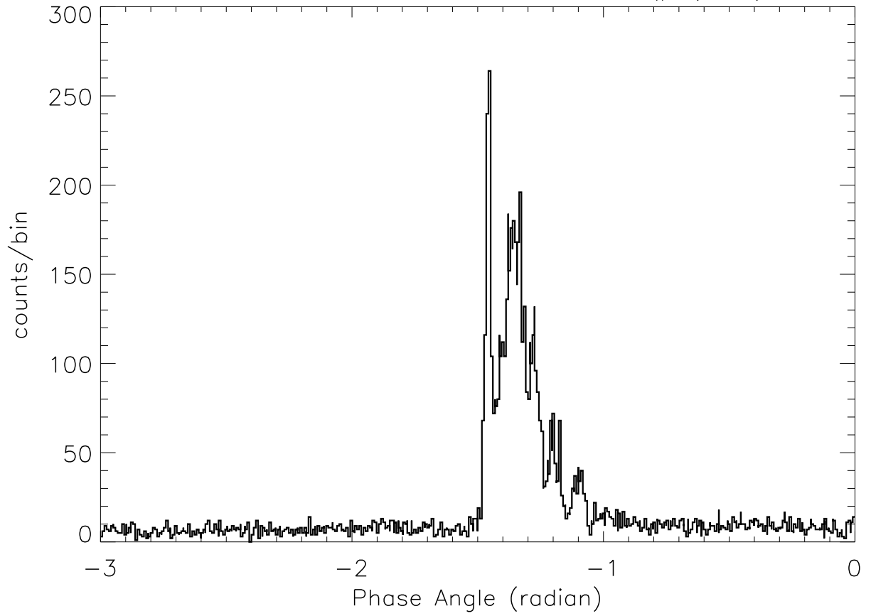
SOX2: 4:40:22 - 4:40:31 SP# ( 62)
