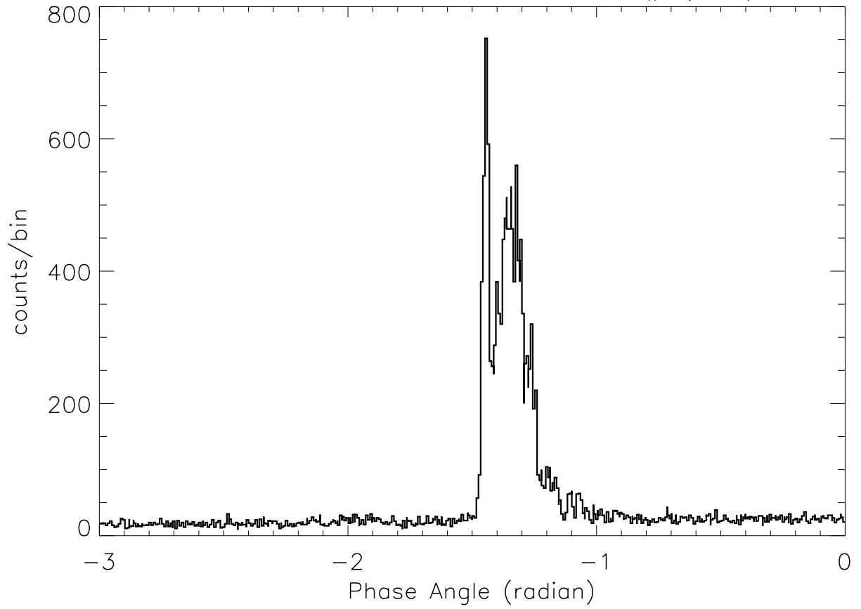
SOX2: 4:37:26 – 4:37:35 SP# ( 42)
