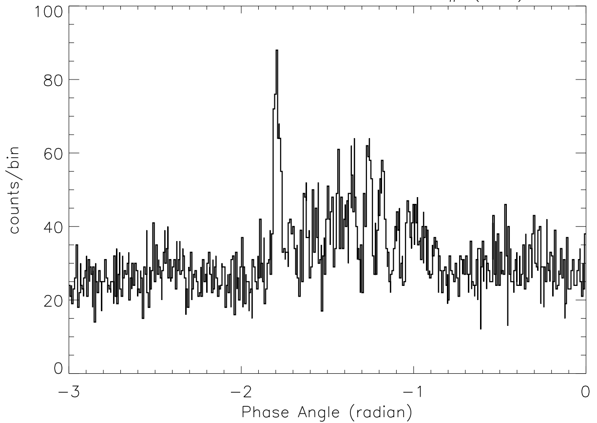
SOX2: 4:38:28 – 4:38:37 SP# ( 49)
