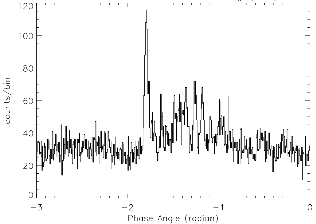
SOX2: 4:38:10 – 4:38:19 SP# ( 47)
