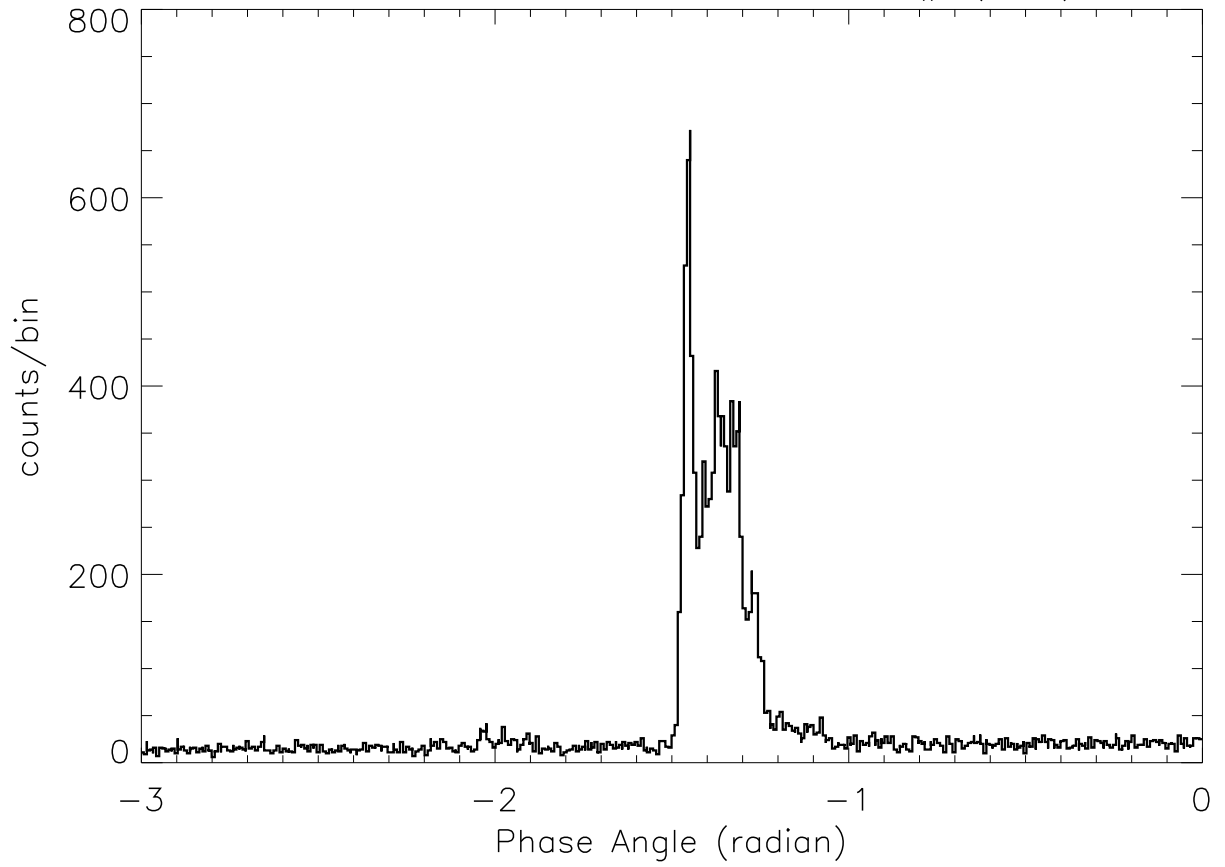
SOX2: 4:34:48 – 4:34:57 SP# ( 24)
