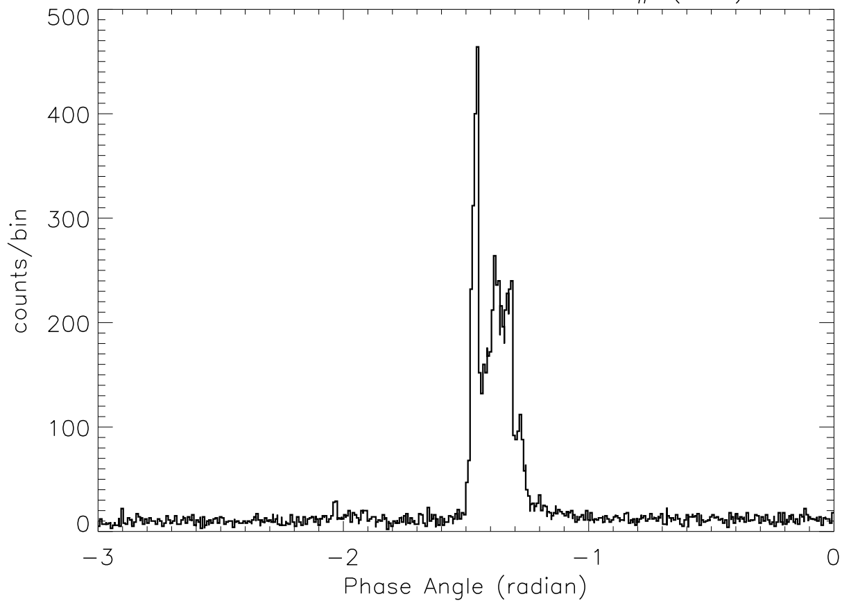
SOX2: 4:34: 4 - 4:34:13 SP# ( 19)
