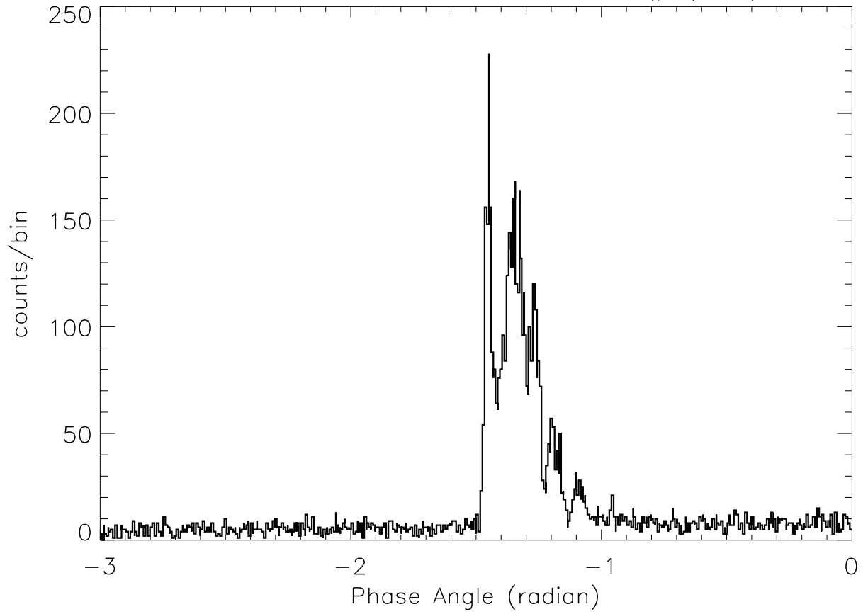
SOX2: 4:41: 6 – 4:41:15 SP# ( 67)
