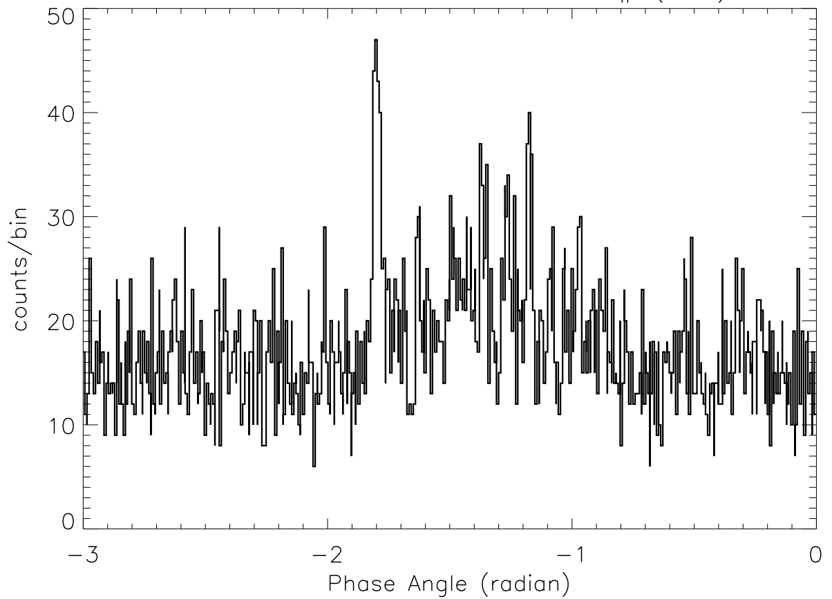
SOX2: 4:40: 5 – 4:40:13 SP# ( 60)
