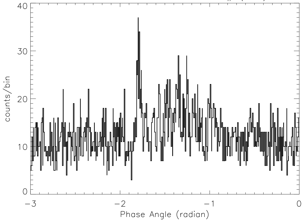
SOX2: 4:41: 6 – 4:41:15 SP# ( 67)
