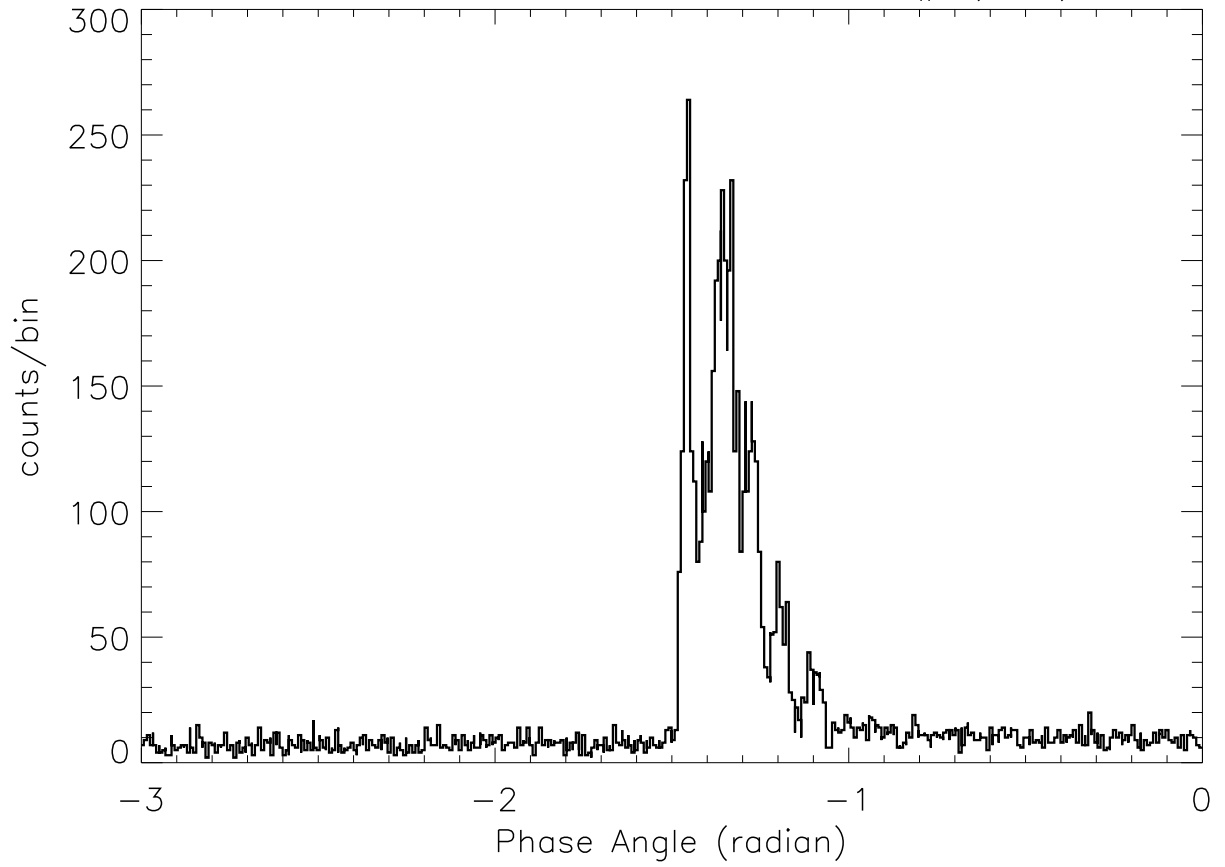
SOX2: 4:40: 5 – 4:40:13 SP# ( 60)
