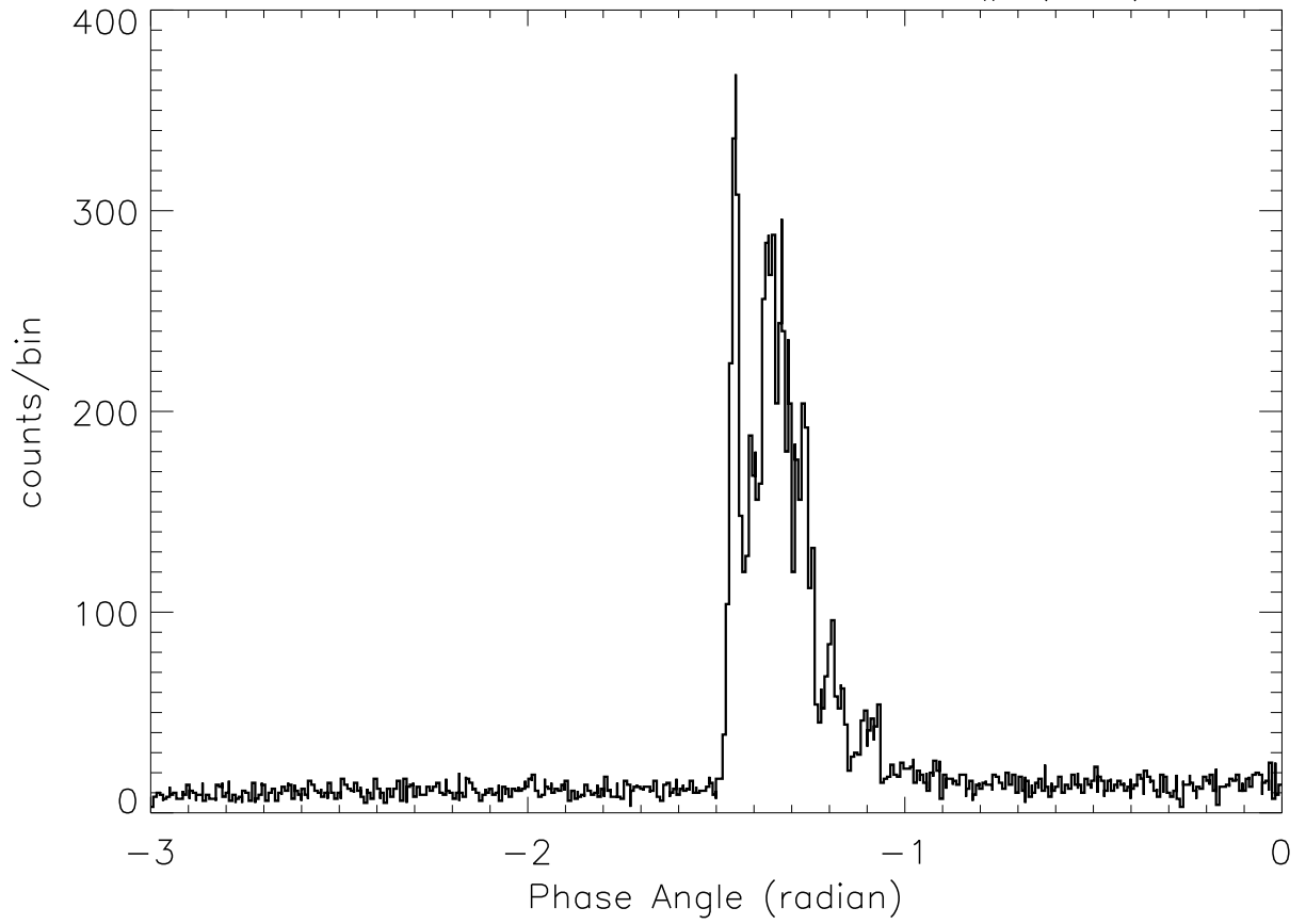
SOX2: 4:39:12 – 4:39:21 SP# ( 54)
