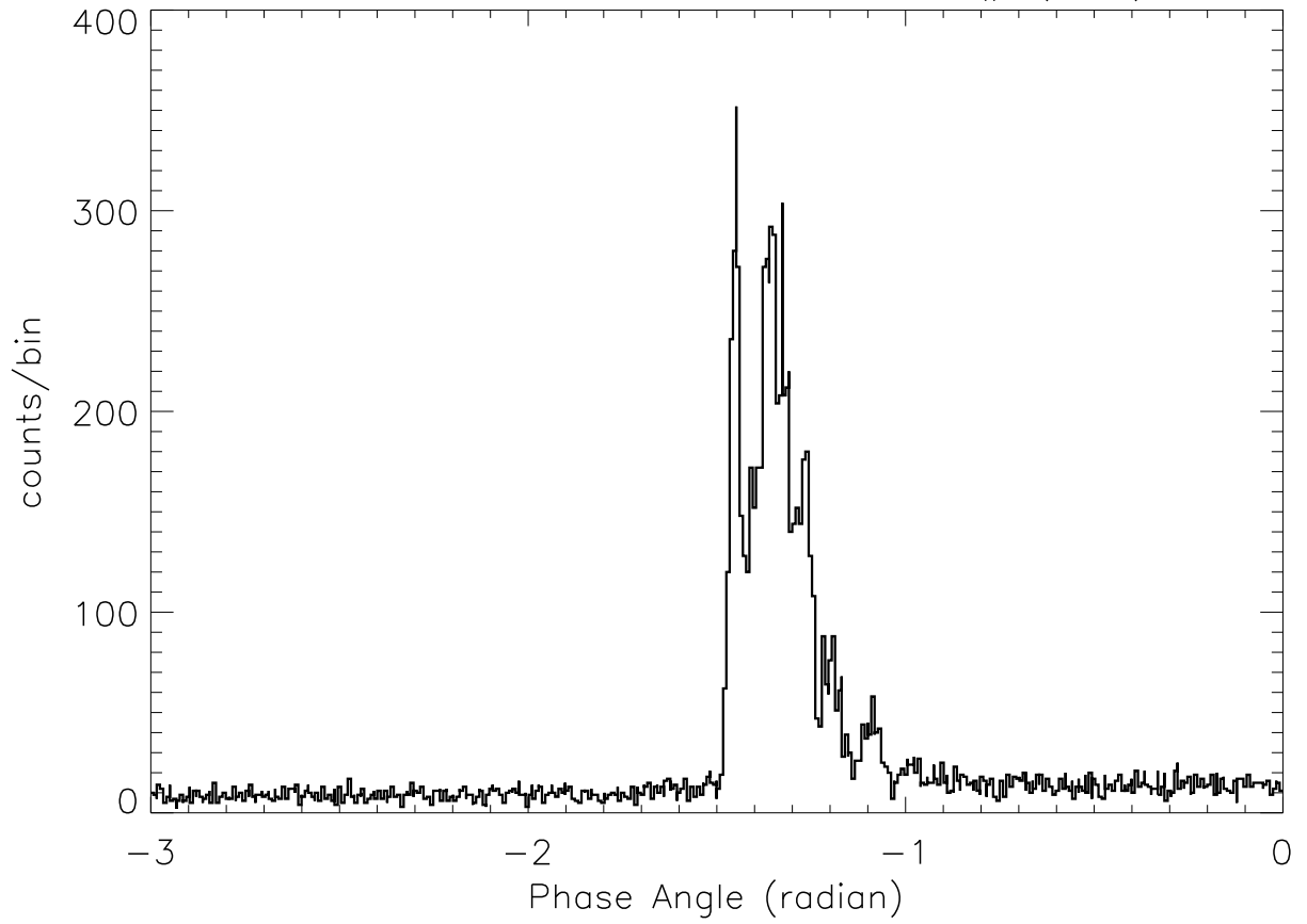
SOX2: 4:39:21 - 4:39:29 SP# ( 55)
