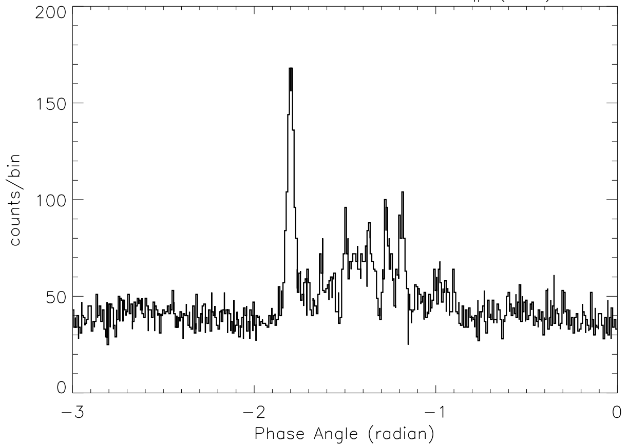
SOX2: 4:36:25 - 4:36:34 SP# ( 35)
